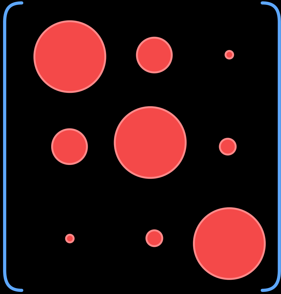
СКМ Matrix
