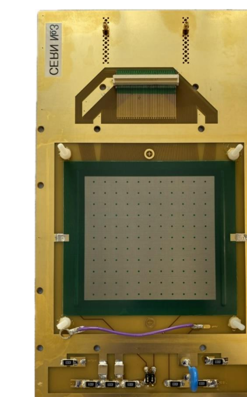
Прототип Micromegas
